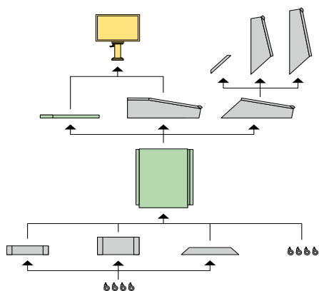
Kombinasjoner med IW deler
